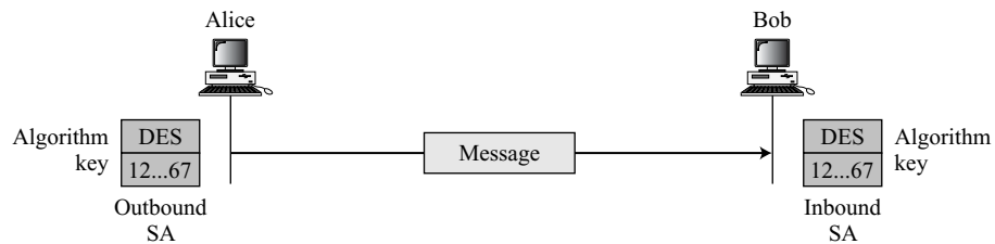
Figure 18.10 Simple SA
